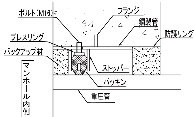
現場打ちマンホール用 取付断面図
