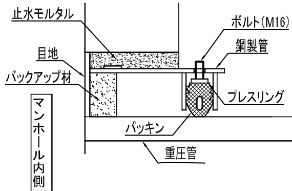
組立てマンホール用 取付断面図
