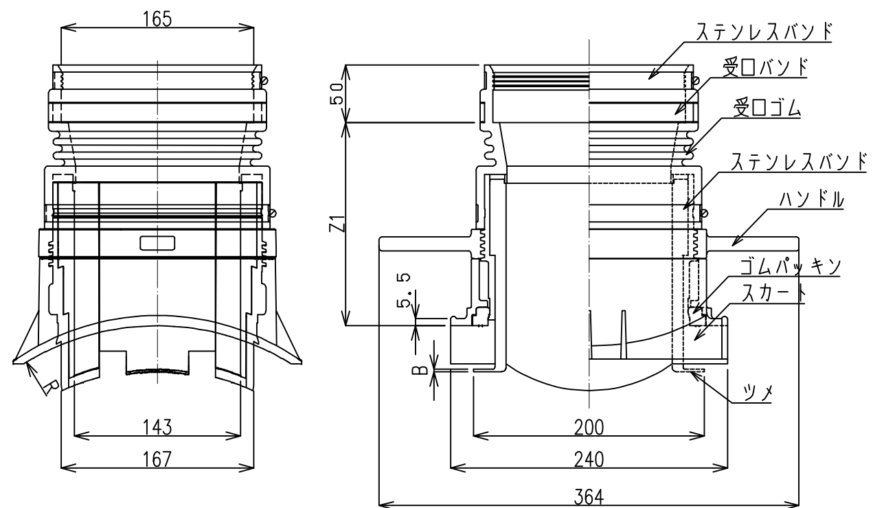
取付管150用
