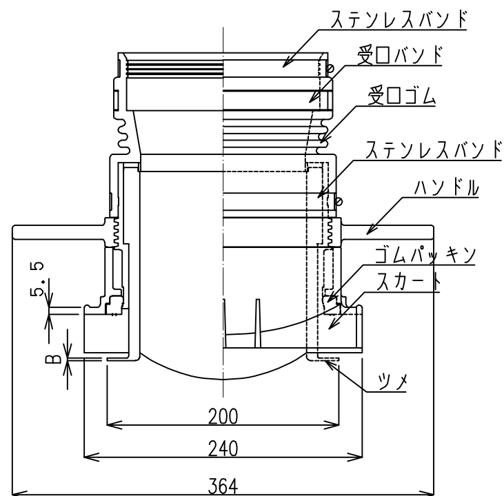
取付管150用
