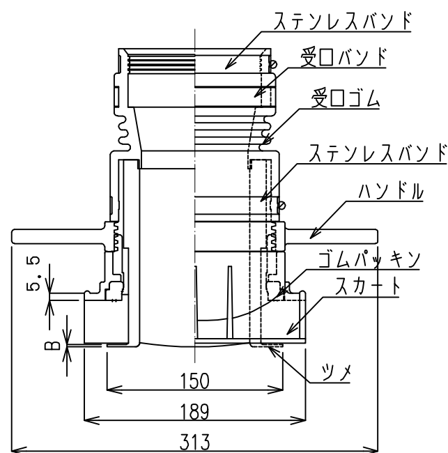
取付管100用
