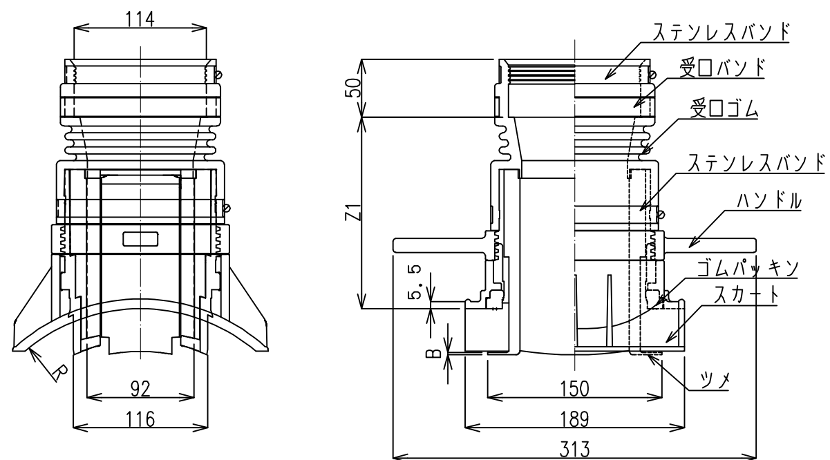
取付管100用
