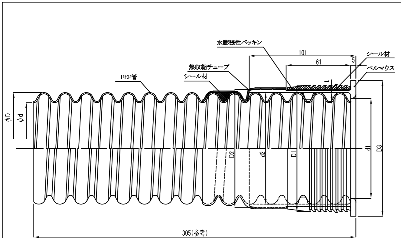
<寸法表>
